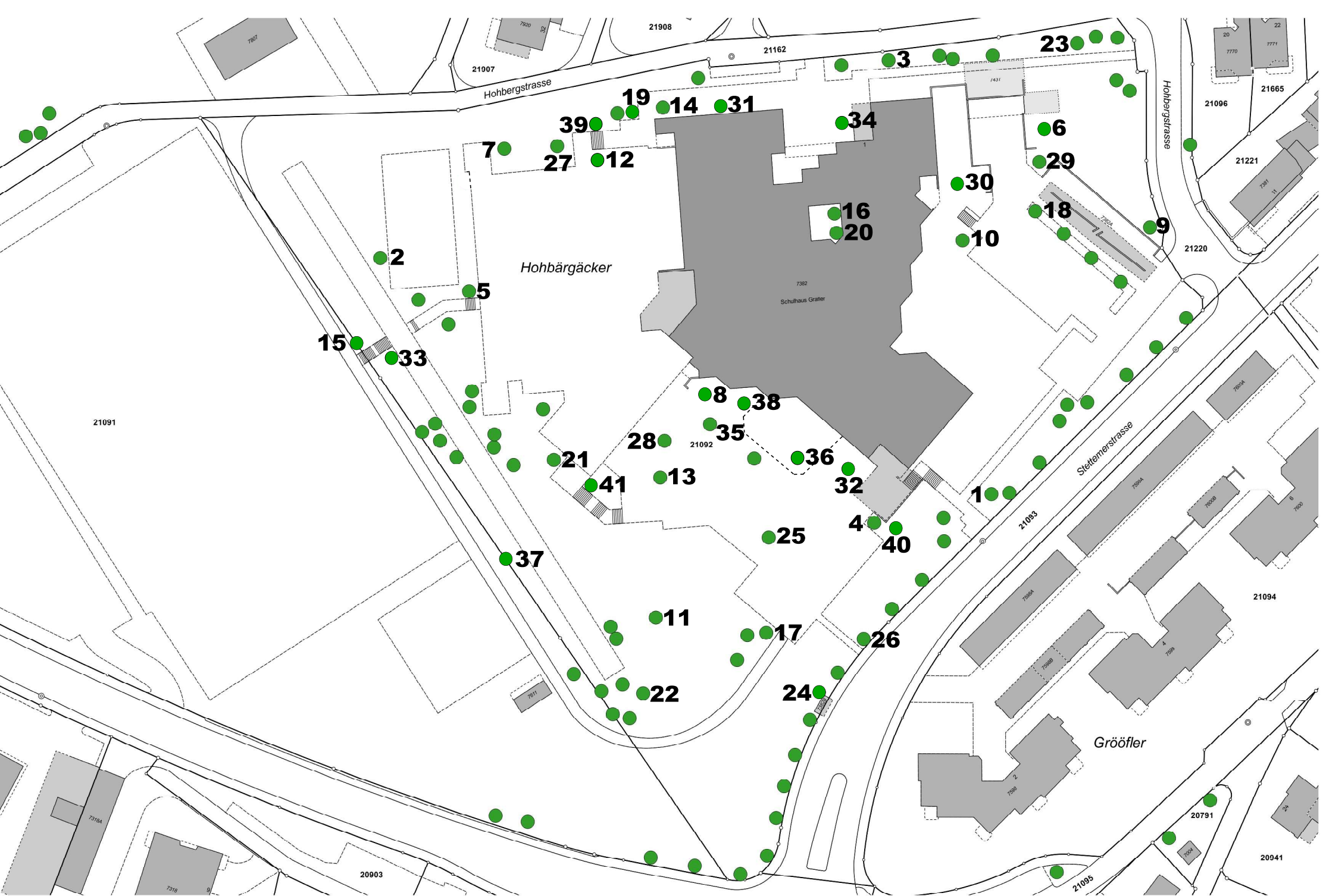
Grün Schaffhausen/Bauminventar
